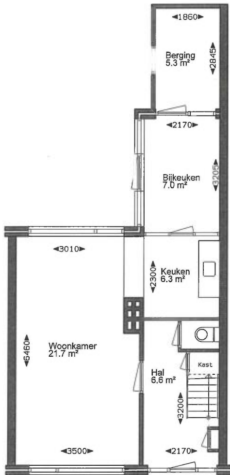
Type 03C Begane Grond
